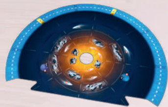
поле Сонячної системи
